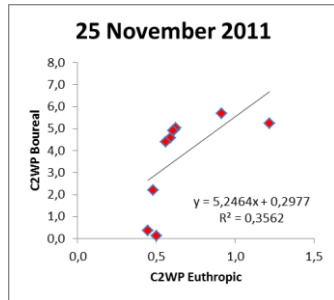
Nilai Relasi C2WP Boureal dan C2WP Euthropic untuk parameter Total Suspended Solid
