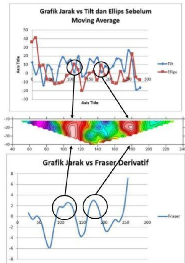
Gambar 2. Korelasi Jarak vs Tilt dan Ellips dengan RAE dan Fraser
