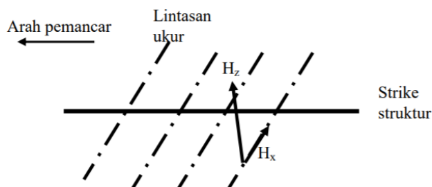
Gambar 1. Pengukuran VLF dengan Mode Tilt-Angle
