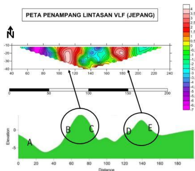
Gambar 3. Hubungan Slope dan Peta RAE (Jepang)
