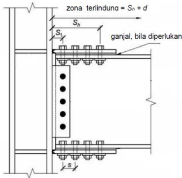
Gambar 3. Sambungan Terpraktualifikasi Tipe PSB
