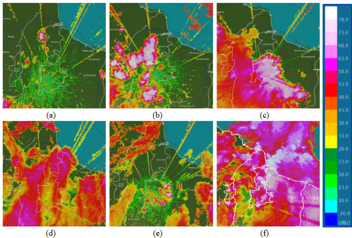
Gambar 3: Hasil Produk VIR pada pukul (a) 12.30 WIB, (b) 13.30 WIB, (c) 15.00 WIB, (d) 17.00 WIB, (e) 18.10 WIB, dan (f) 22.00 WIB.
