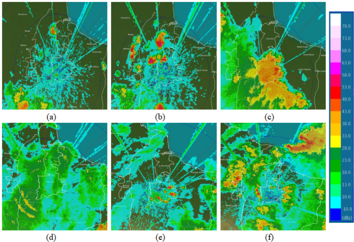
Gambar 2: Hasil Produk CMAX pada pukul (a) 12.30 WIB, (b) 13.00 WIB, (c) 15.00 WIB, (d) 17.00 WIB, (e) 18.10 WIB, dan (f) 20.30 WIB.
