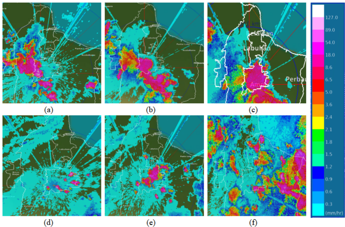
Gambar 4: Hasil Produk CMAX momen intensitas curah hujan rata-rata pada pukul (a) 14.00 WIB, (b) 14.30 WIB, (c) 15.00 WIB, (d) 18.10 WIB, (e) 18.30 WIB, dan (f) 21.10 WIB.
