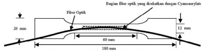
Gambar 2: Ukuran dan bentuk spesimen uji A5052 Aluminium Alloy
