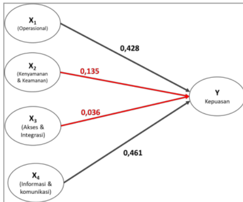
Gambar 4. Diagram Jalur Akhir
