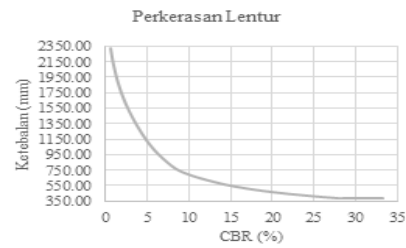
Gambar 3. Grafik tebal perkerasan lentur.
