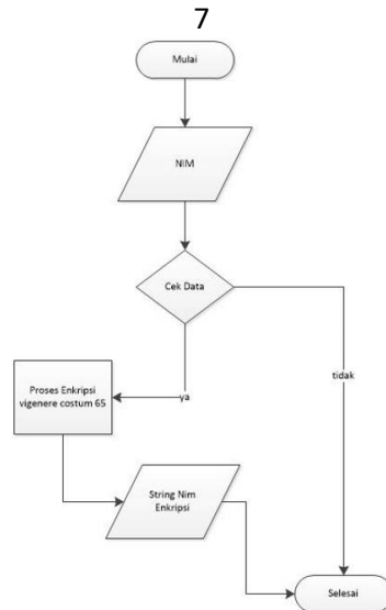
Gambar 12 Proses Enkripsi
